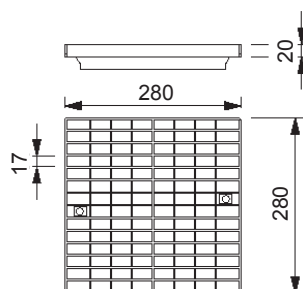
Ocelový pozinkovaný rošt kN B 125
